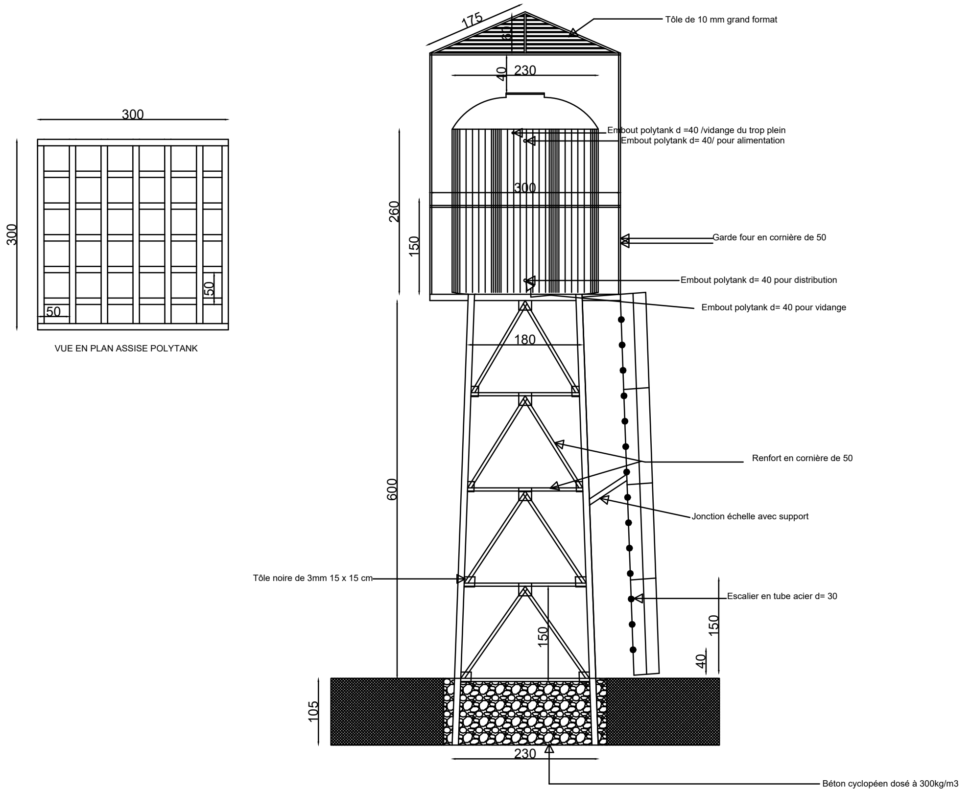
VUE EN PLAN D'UN SUPPORT METALLIQUE AVEC UN POLYTANK DE 10 m3
